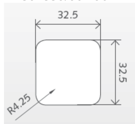
SCASSO/CUT OUT
