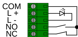
CIRCUITO INTERNO "JP2"
