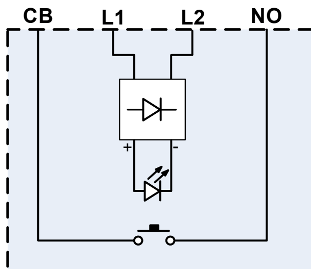
Schema di collegamento / wiring diagram
