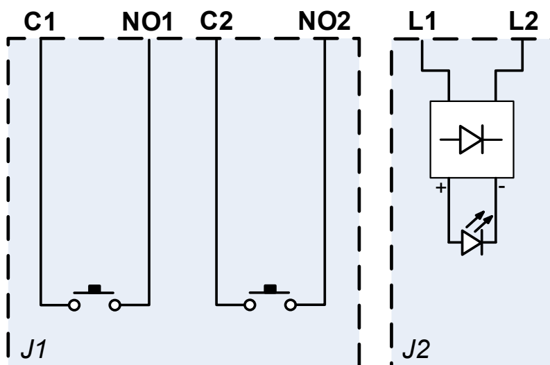
Schema di collegamento / wiring diagram
