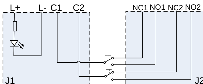
Schema di collegamento/ wiring diagram
