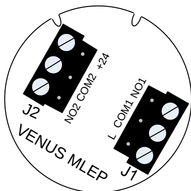
Morsetto estraibile/ extractable terminal: 5.08mm
