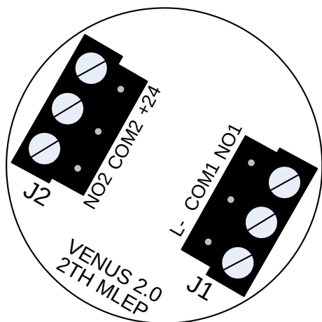
Morsetto estraibile/ extractable terminal: 5.08mm
